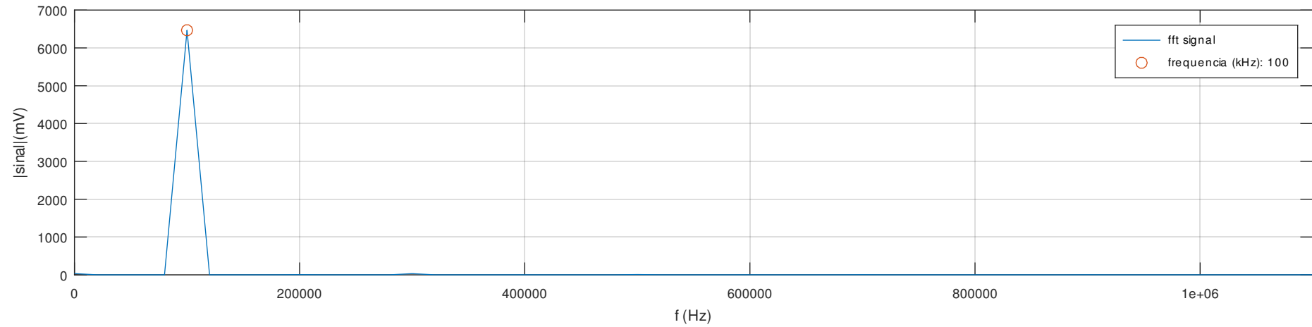
Espectro de amplitudes unilateral X(t) - Saída f=100\text{kHz} do gerador de sinais com ganho máximo
